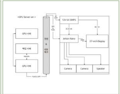
▲ 제품 설계도 - jetson Nano Pinout-GPU서버 사용 시
